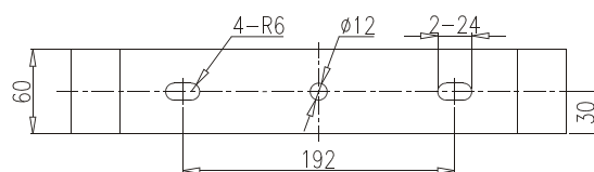
U型支架安装孔位
