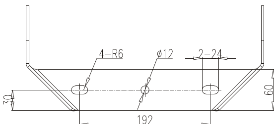
折弯支架安装孔位
